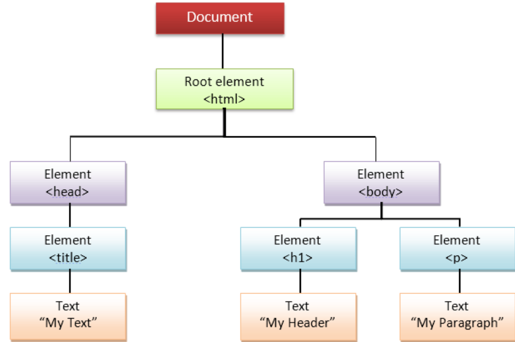
DOM Tree(Real)
